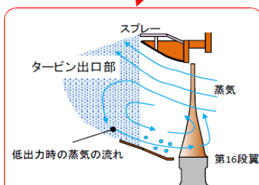
図1 スプレーの水滴による翼の浸食
