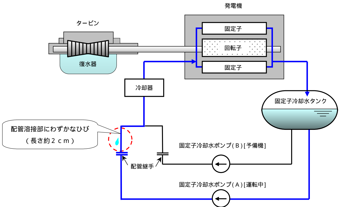
志賀原子力発電所 2号機 発電機固定子冷却系概略図
