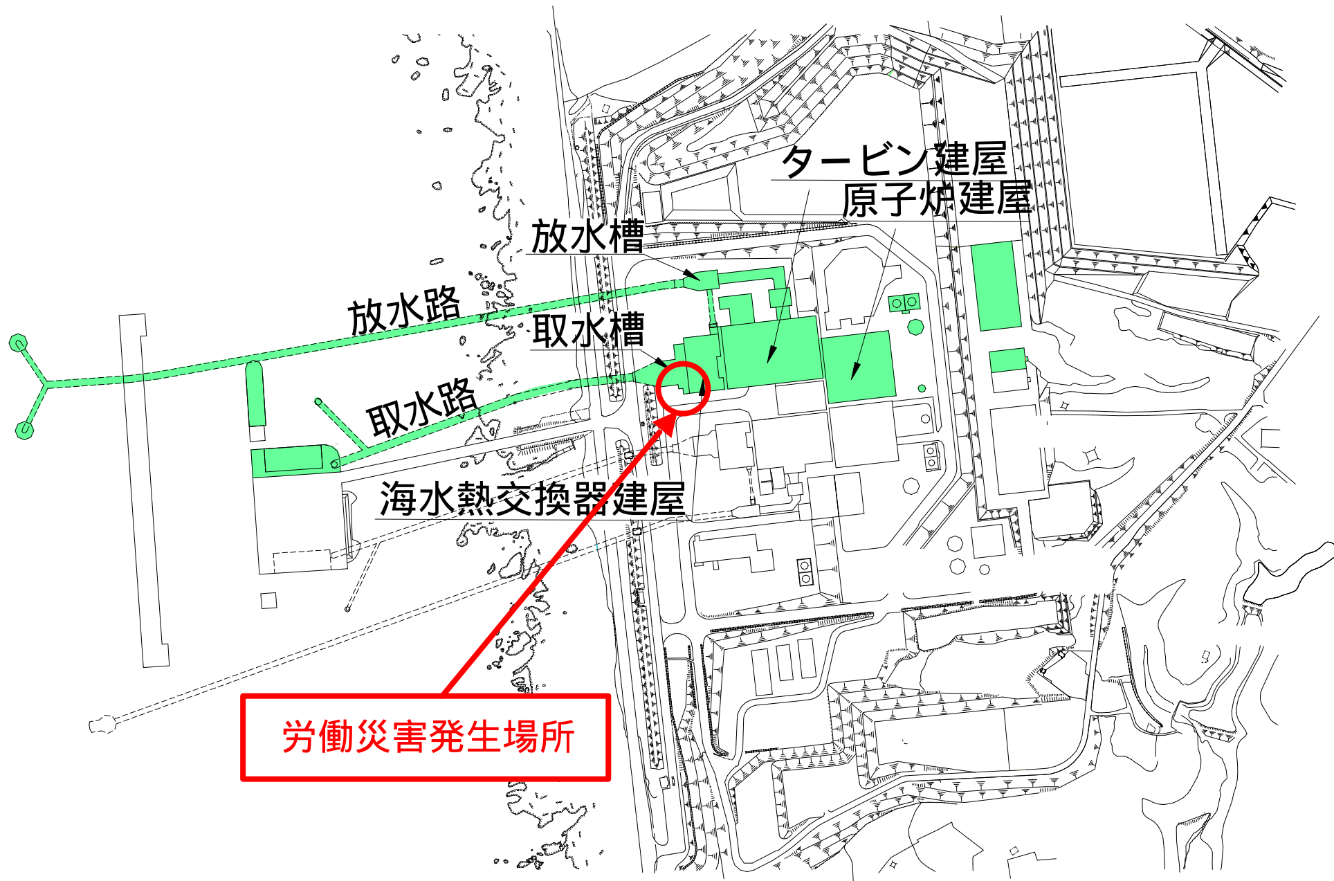
< 志賀原子力発電所 2号機建設工事エリア概要図 >
