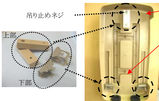
嵩上げ具の開発
