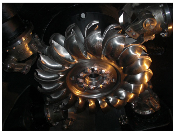
称名川第二発電所 水車羽根車（ランナ）
